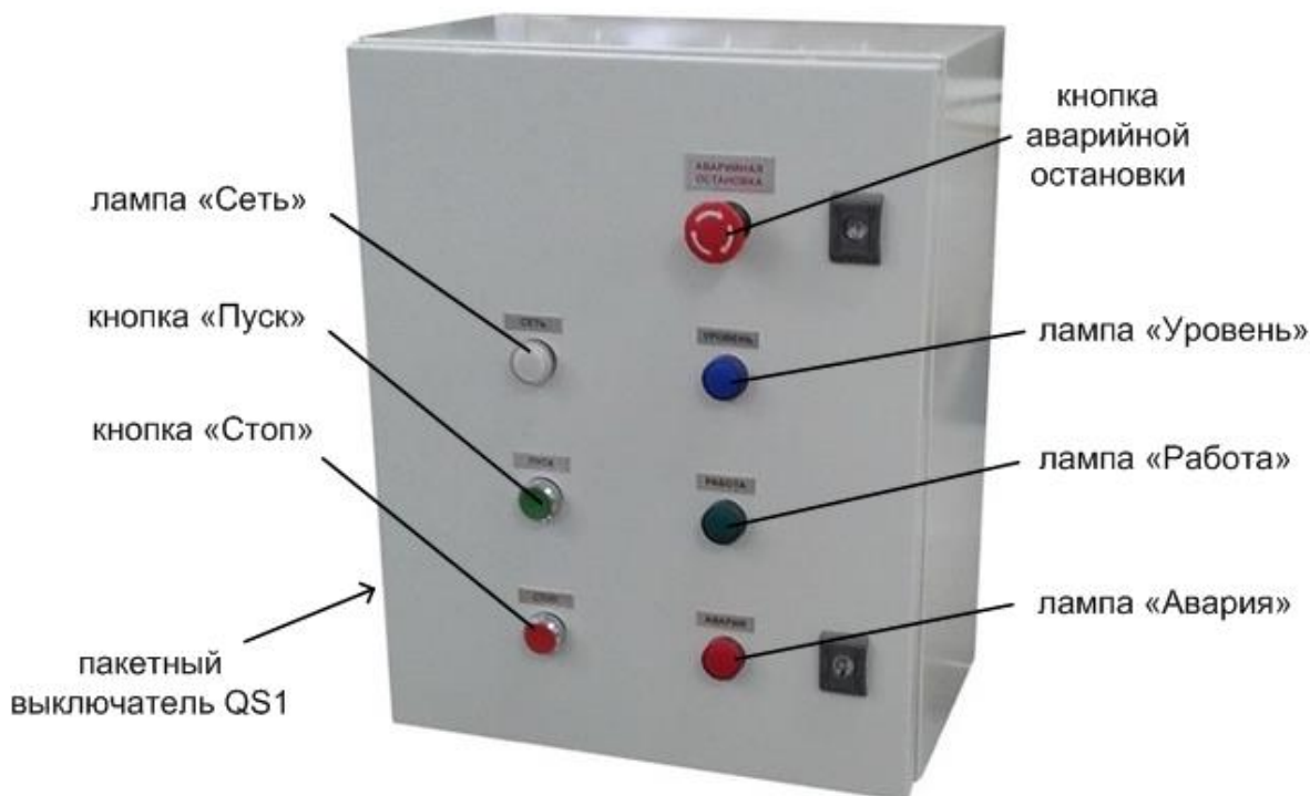
Рис.4 Блок управления.
