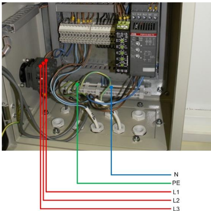
Рис.7 Подключение электропитания.
