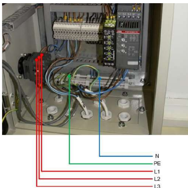
Рис.7 Подключение электропитания.
