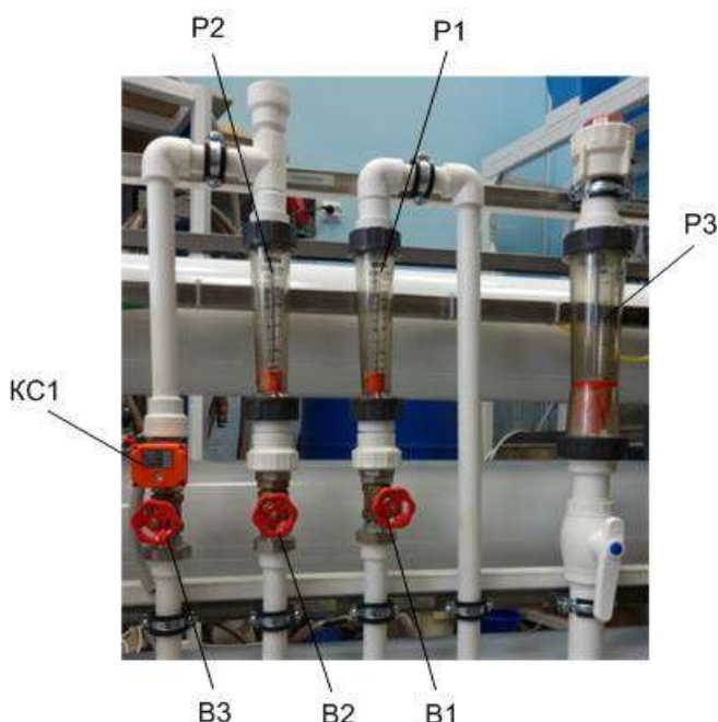
Рис.3 Ротаметры и вентили
