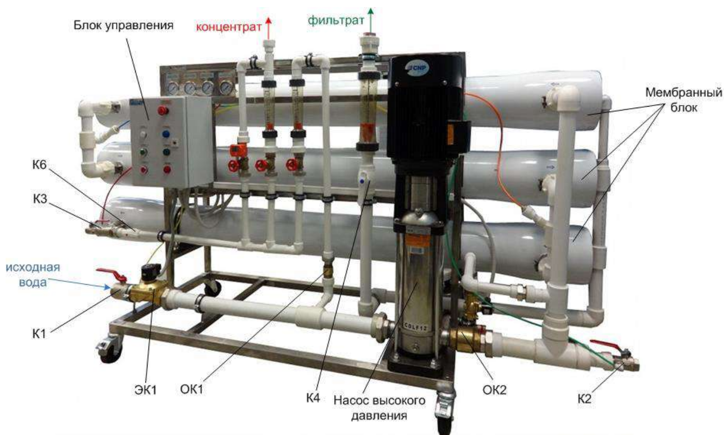
Рис.1 Общий вид установки.
