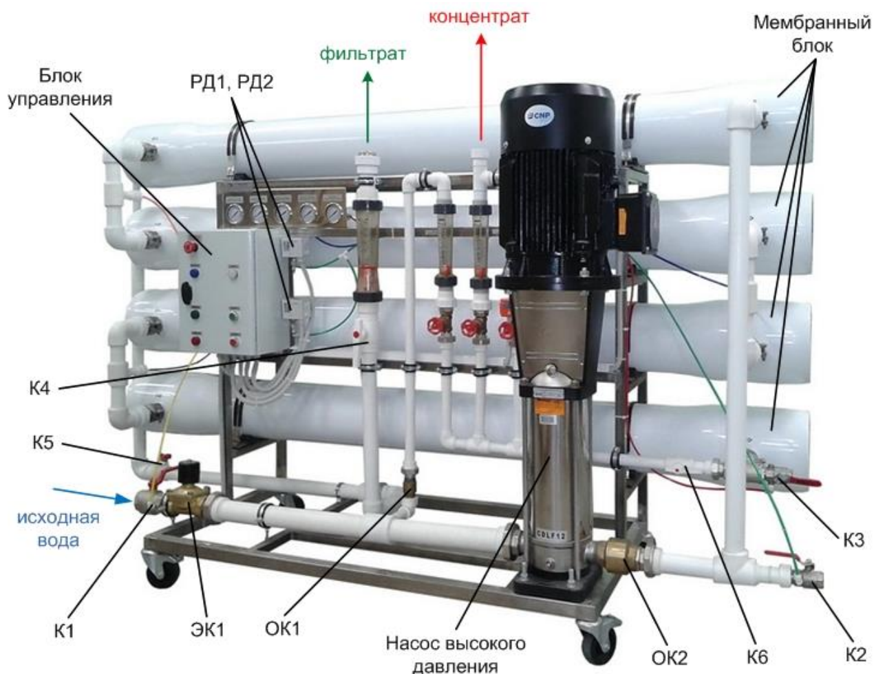
Рис.1 Общий вид установки.
