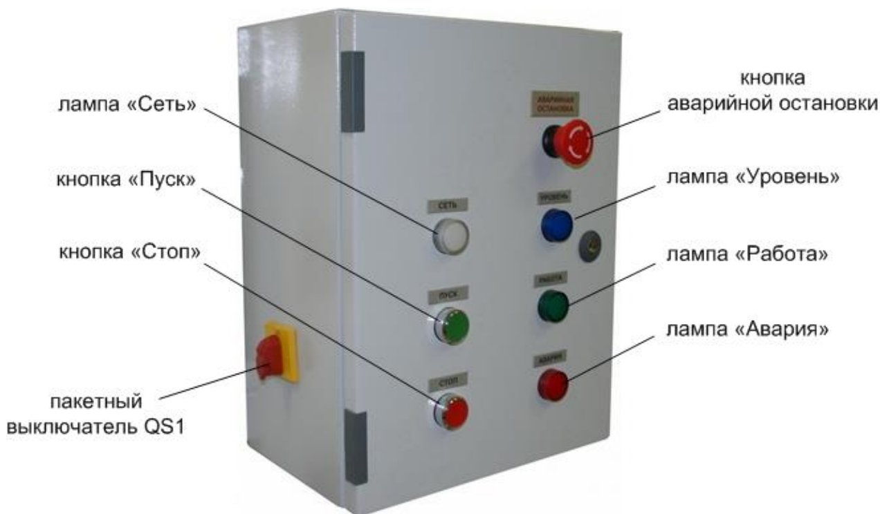
Рис.4 Блок управления.
