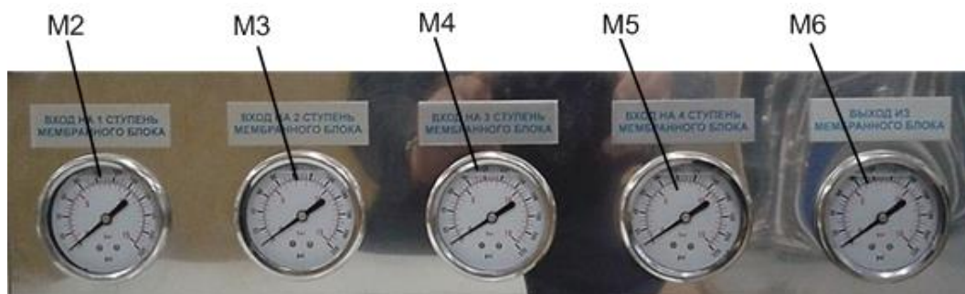
Рис.2 Панель манометров.
