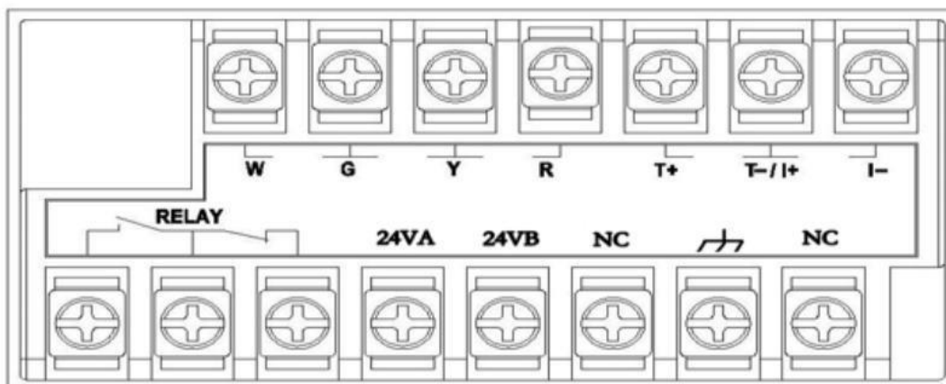
Исполнение 24В
