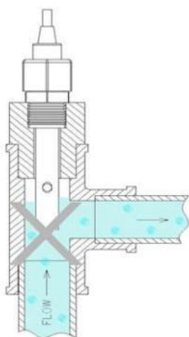
Неправильная
