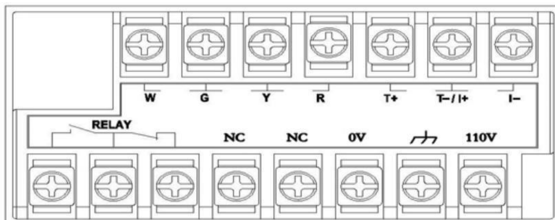
Исполнение 110В
