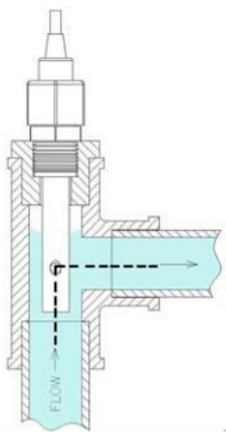
Правильная
