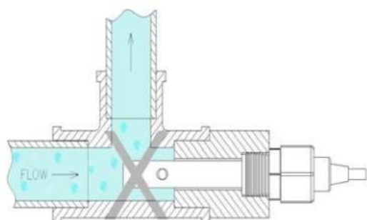
Неправильная
